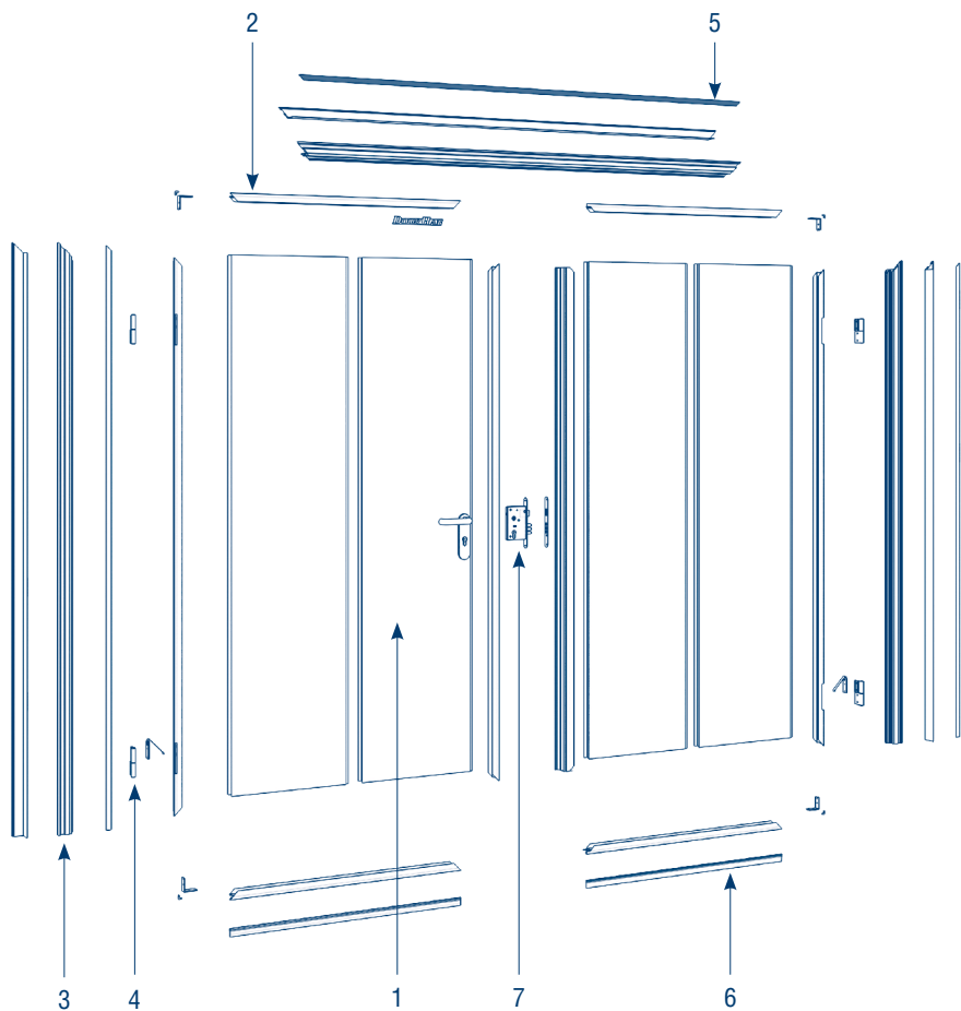
Рис. 1. Конструкция дверей
